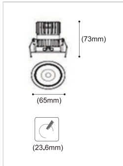
SIZE | LED-D512-7W
